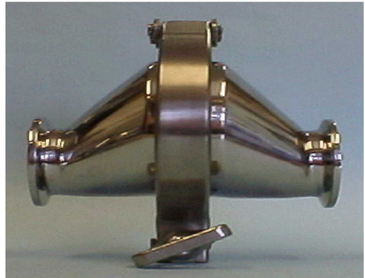
接続部:IDF1.5Sヘルレル エレメント部:IDF3Sヘルレル
