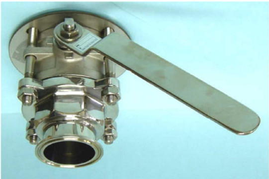
接続部:IDF2Sヘルール ボトムフランジ無し
